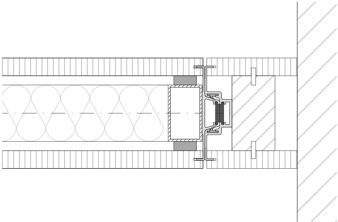
Wandanschluss Normalelement
